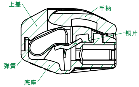
剖面
